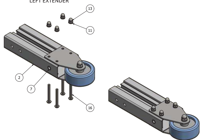
LEFT EXTENDER
