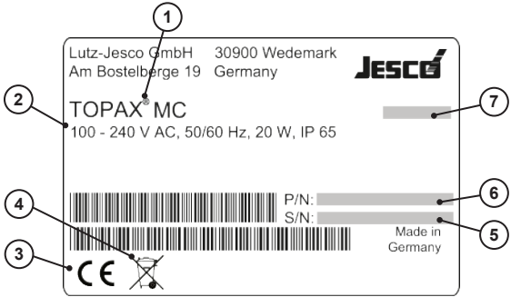
Figur 6: Typebetegnelse flerkanaals regulator TOPAX® MC
