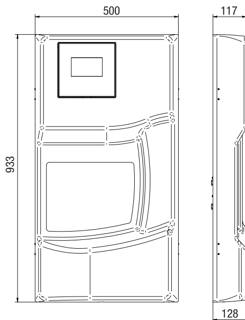
Figur 10: Dimensioner afdækningshætte målevandspaneler EASYPRO 3, 4, MC-C, MD-C, MP-C
