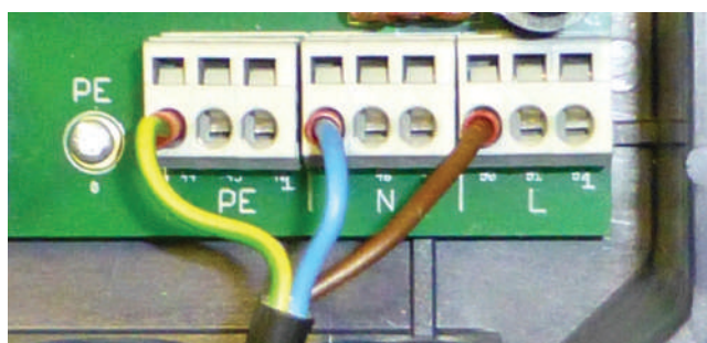
Figur 14: Tilsluttet strømforsyning
