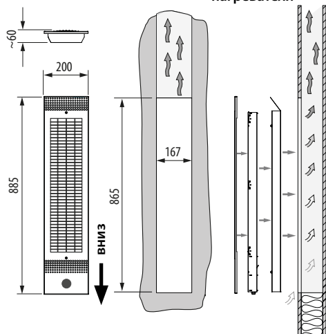
Вырез в стене с вентиляцией сзади нагревателя
